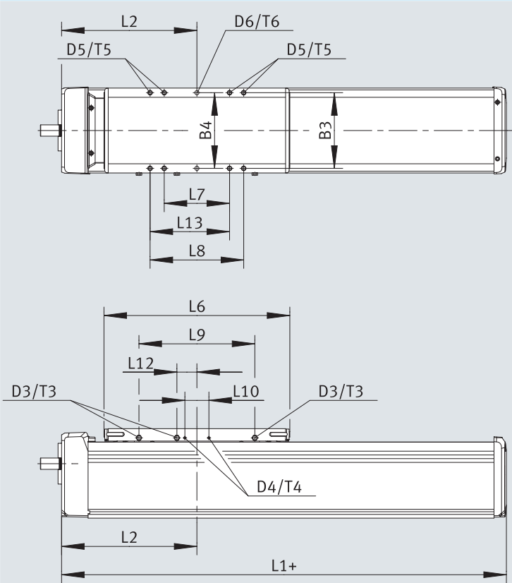
外形寸法図 - ELGD-BS-120_-L(ロングテーブル)
