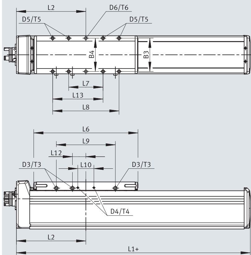
外形寸法図 - ELGD-BS-60/80_-L(ロングテーブル)
