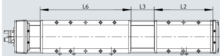
外形寸法図 - ELGD-BS-_-ZR(追加テーブル)
