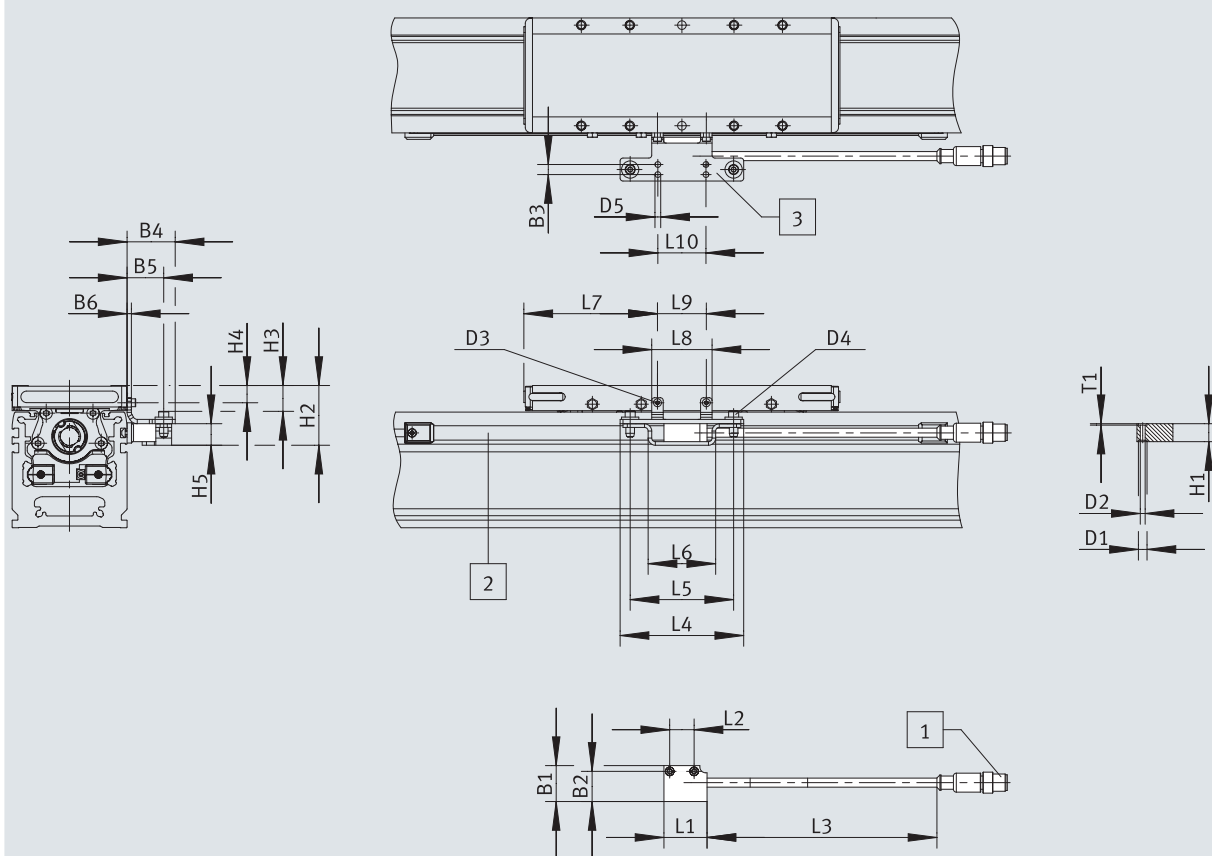
外形寸法図 - ELGD-_-M3 エンコーダ付
