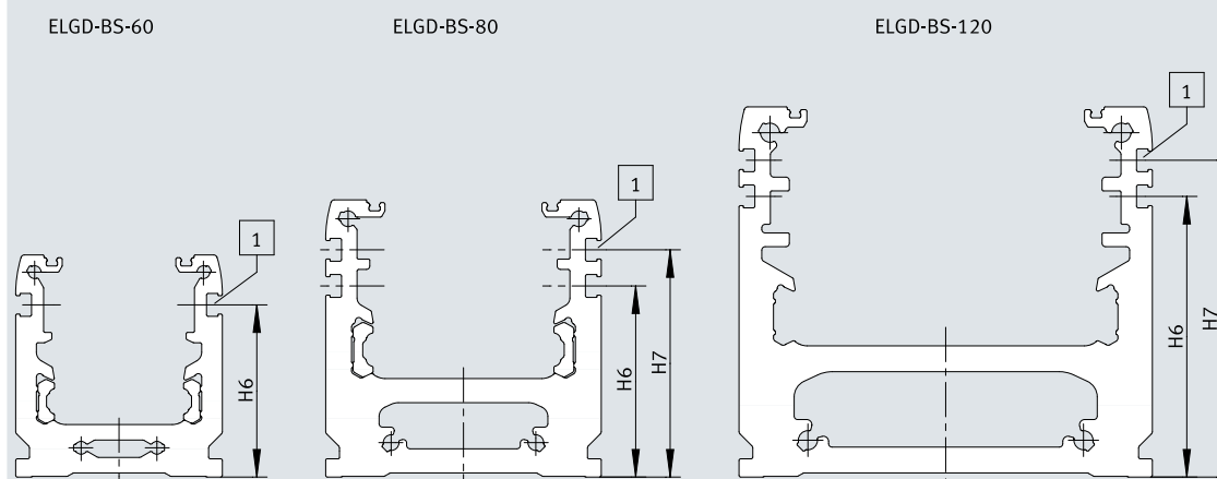
外形寸法図 - ELGD-BS-_- (フレーム)
