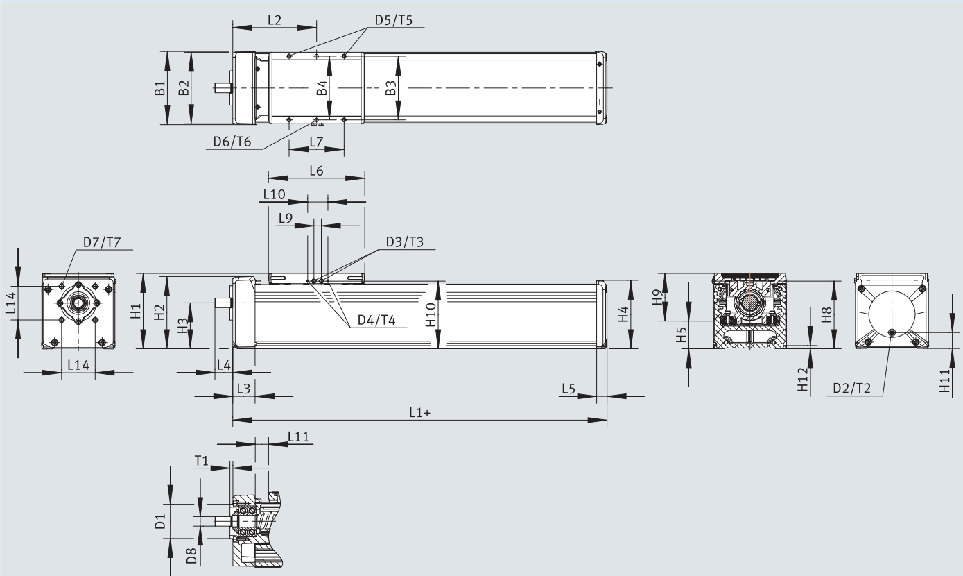
外形寸法図 - ELGD-BS-120_
