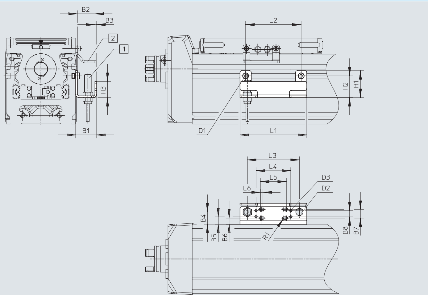
外形寸法図 - センサブラケット EAPM-E24-60-SHO
