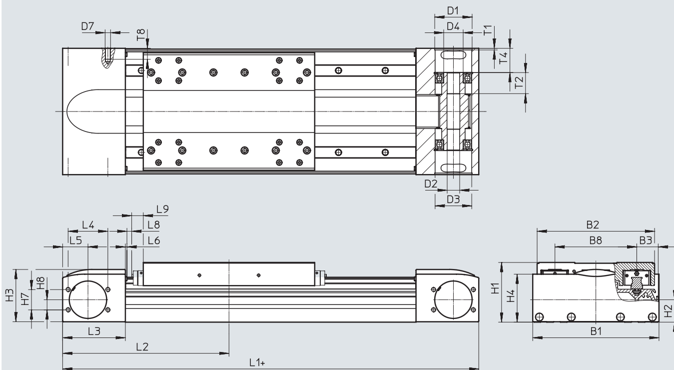
外形寸法図
