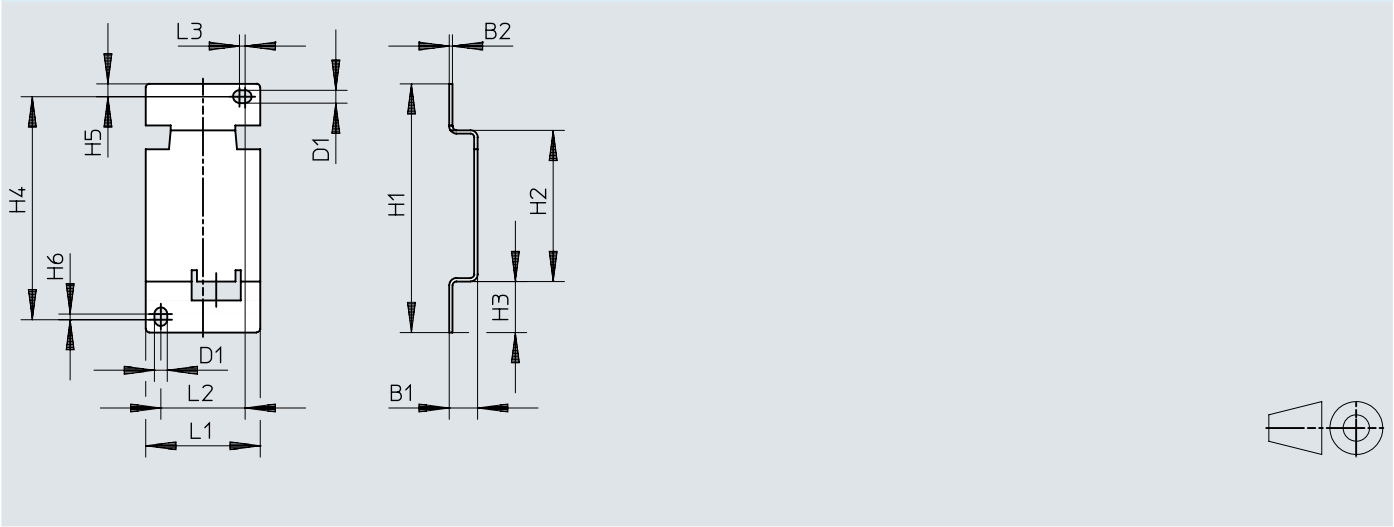
Dimensioni – Piastra di adattamento SDE1- ...-W ...
