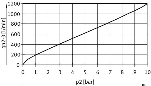
Caudal qn de 2 -> 3 en función de la sobrepresión de salida p2, VPPM-6L/F-...-0L10H-... (10 bar)
