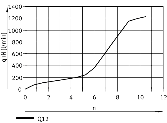
Caudal nominal normal qnN a 0,6 → 0,5 MPa en función de las revoluciones del husillo n para la unión roscada G1/2, R1/2 (aire de escape)
