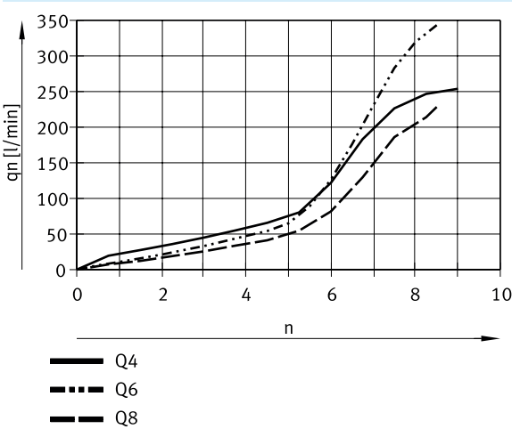
Caudal normal qn a 0,6 → 0 MPa en función de las revoluciones del husillo n para la unión roscada G1/8, R1/8 (aire de escape)
