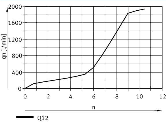
Caudal normal qn a 0,6 → 0 MPa en función de las revoluciones del husillo n para la unión roscada G1/2, R1/2 (aire de escape)
