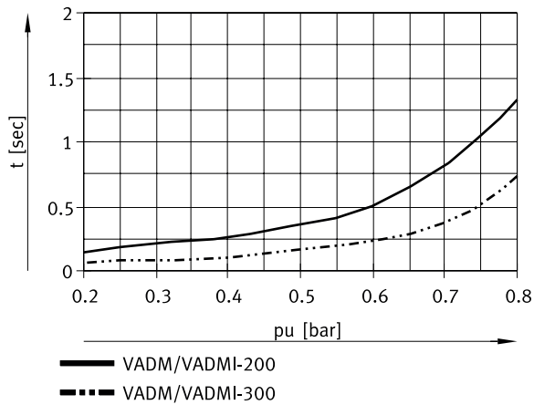
Tiempo de evacuación t [s] para 1 litro de volumen con presión de funcionamiento de 6 bar (anchura nominal de la boquilla Laval 200/300)
