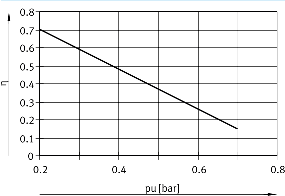
Rendimiento \eta en función del vacío \Delta p_u con P_{nom} de 6 bar
