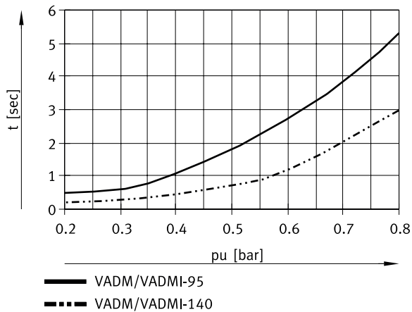
Tiempo de evacuación t [s] para 1 litro de volumen con presión de funcionamiento de 6 bar (anchura nominal de la boquilla Laval 95/140)
