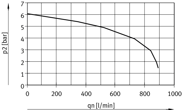
Caudal qn en función de la presión de salida p2 en placas reguladoras de presión (de 20 mm de ancho) (placas de regulación A) para conexiones 4 (placas de regulación B, rev.) para conexiones 3, reversible
