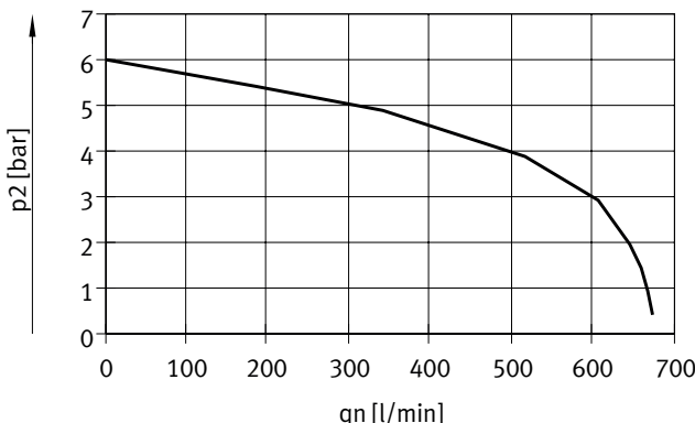
Caudal qn en función de la presión de salida p2 en placas reguladoras de presión (de 20 mm de ancho) (placas de regulación A, rev.) para conexiones 5, reversible
