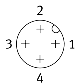
Vista del conector M12, con codificación A
