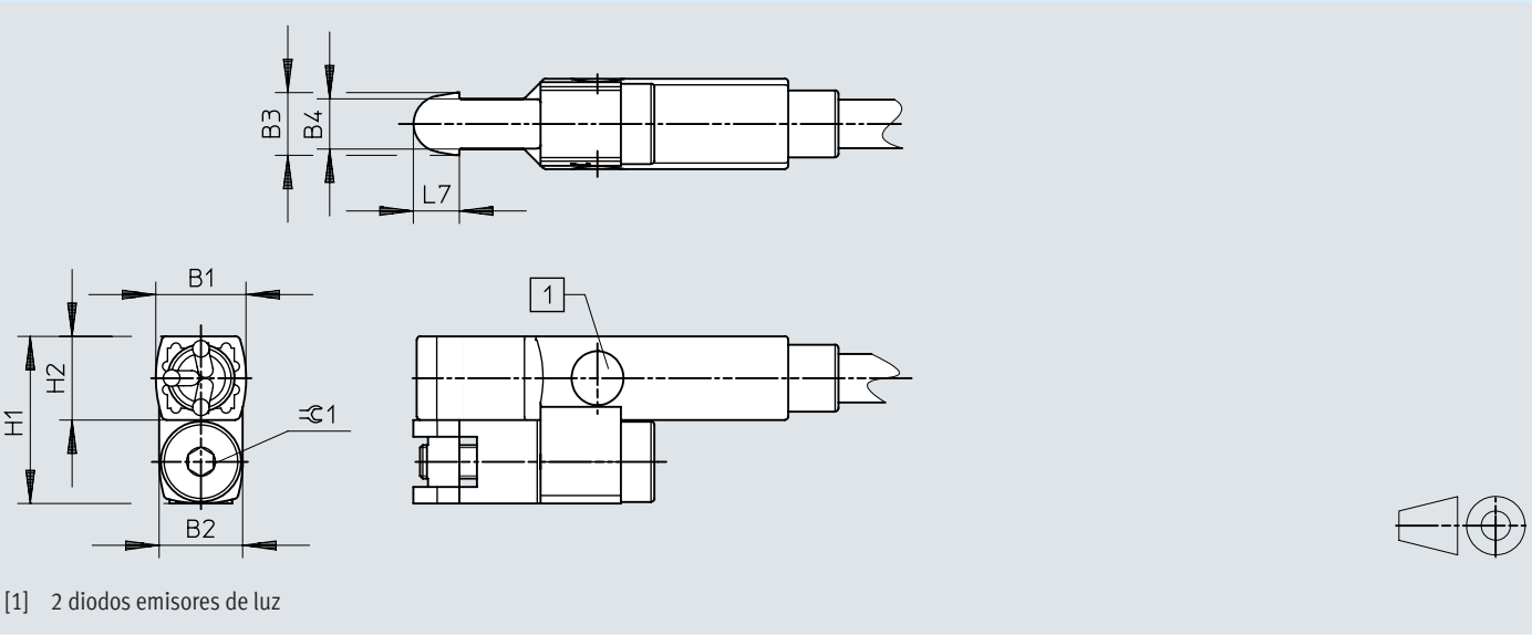
Dimensiones – SMT-10G
