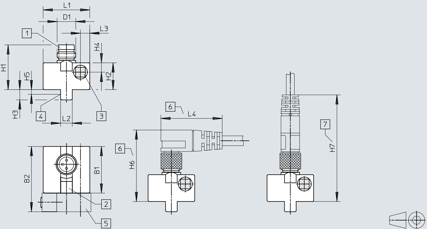
Dimensiones – SMT0-8E-...-S-LED-24 – Stecker M8x1
