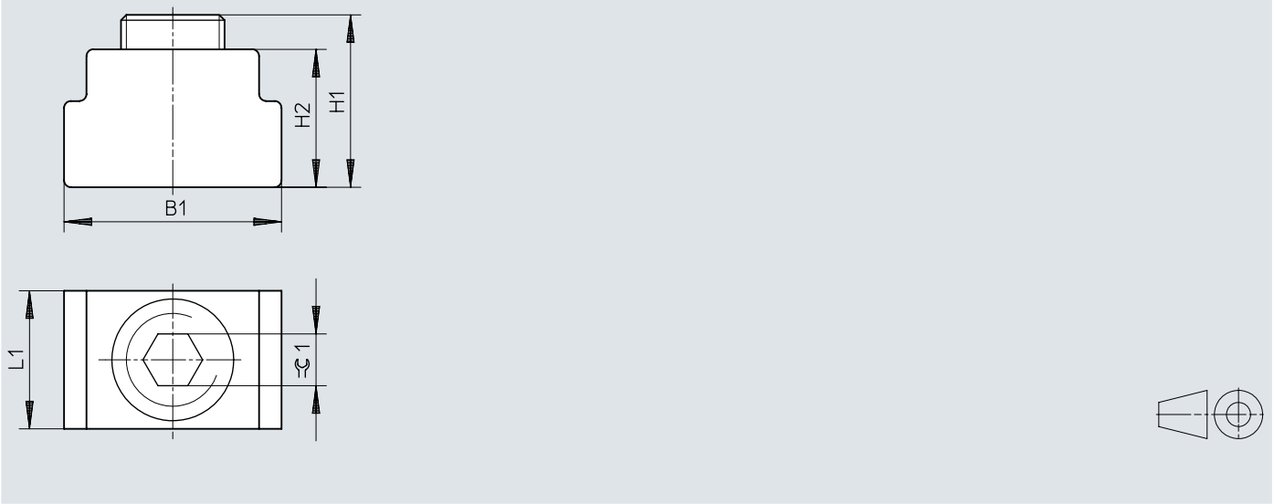
Dimensiones – Elemento de posicionamiento SMM
