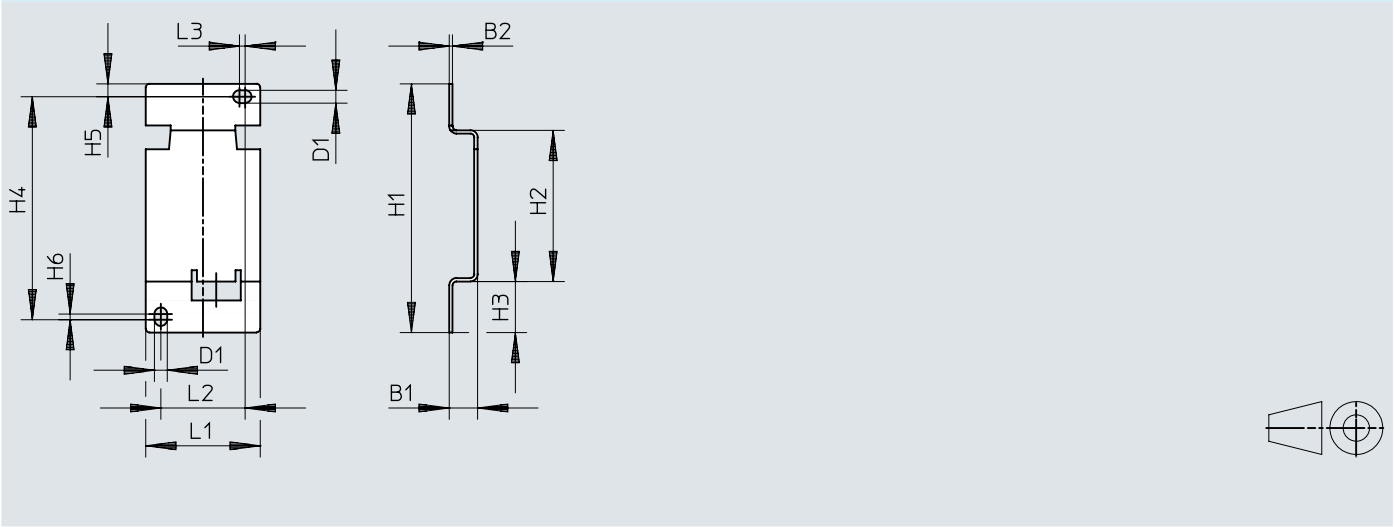
Dimensiones – Placa adaptadora SDE1-...-W ...
