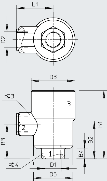
Dimensiones – Conexión neumática G3/8, SEU
