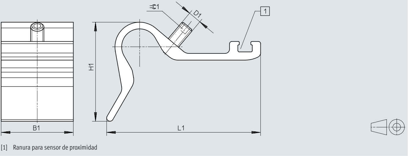
Dimensiones – Soporte para sensor DASP-M4-...-A
