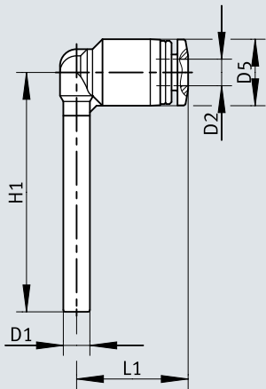
Dimensiones – Racor rápido acodado QSL-...HL-U
