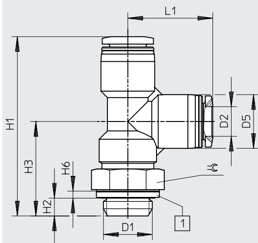
Dimensiones – Racor rápido roscado en T QSTL, rosca G con anillo de junta
