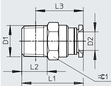
Dimensiones – Racor rápido roscado QS-...-I, rosca R
