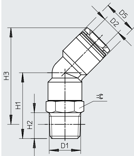
Dimensiones – Racor rápido roscado QSW, rosca R
