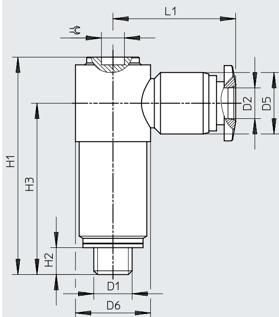
Dimensiones – Racor rápido roscado en L (largo) QSMLLV-...-I
