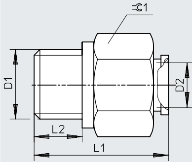
Dimensiones – Racor rápido roscado QSM, rosca G con anillo de junta
