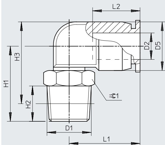
Dimensiones – Racor rápido roscado en L QSML, rosca R
