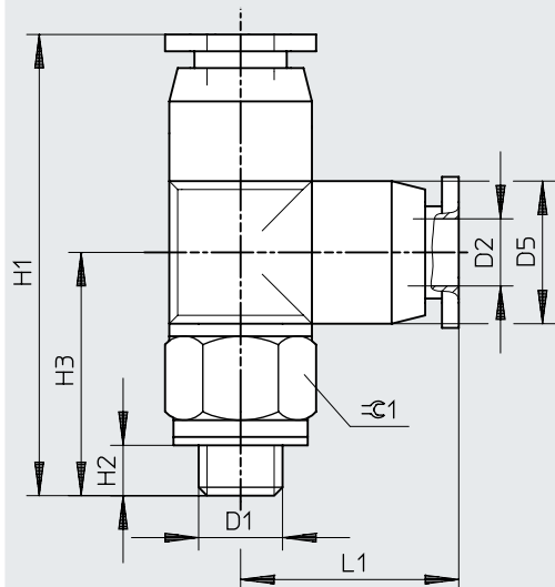
Dimensiones – Racor rápido en T QSMTL, rosca métrica con anillo de junta
