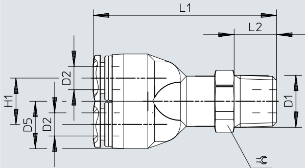
Dimensiones – Racor rápido roscado en Y QBY
