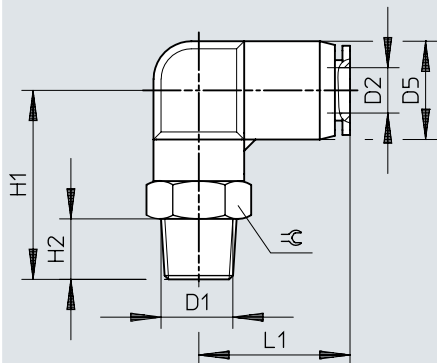
Dimensiones – Racor rápido roscado en L QBL
