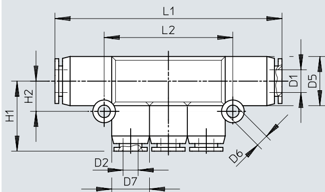
Dimensiones – Distribuidor múltiple QBT3-...T
