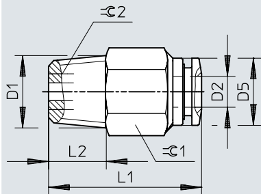
Dimensiones – Racor rápido roscado QB
