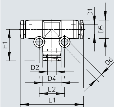
Dimensiones – Unión en T QBMT-...T, reductora
