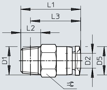
Dimensiones – Racor rápido roscado QBM, rosca NPT
