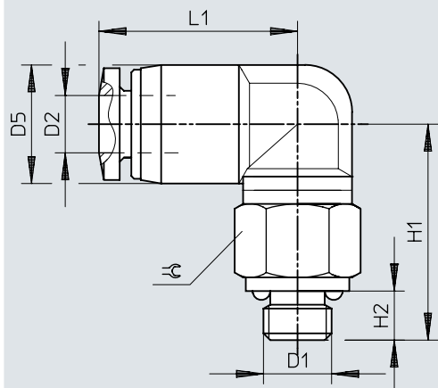
Dimensiones – Racor rápido roscado en L QBML, rosca UNF
