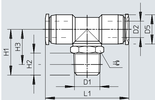
Dimensiones – Racor rápido en T QBMT, rosca NPT
