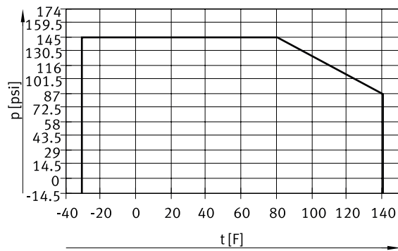
Presión de funcionamiento p en función de la temperatura t (PUN-H; NPT)
