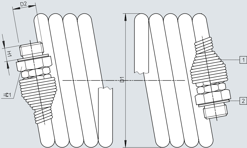
Dimensiones – Tubo de plástico espiral PPS
