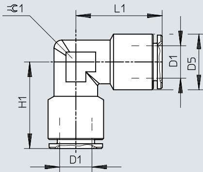
Dimensiones – Racor rápido acodado NPQML
