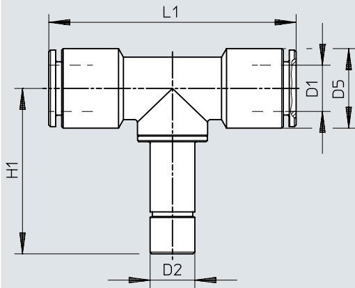
Dimensiones – Unión en T NPQM-T con casquillo enchufable
