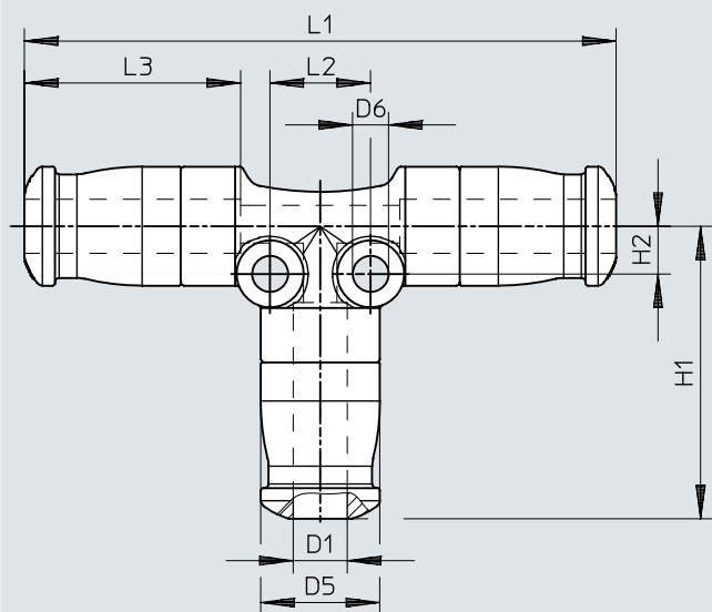
Dimensiones – Conexión en T encastrable NPKA-T
