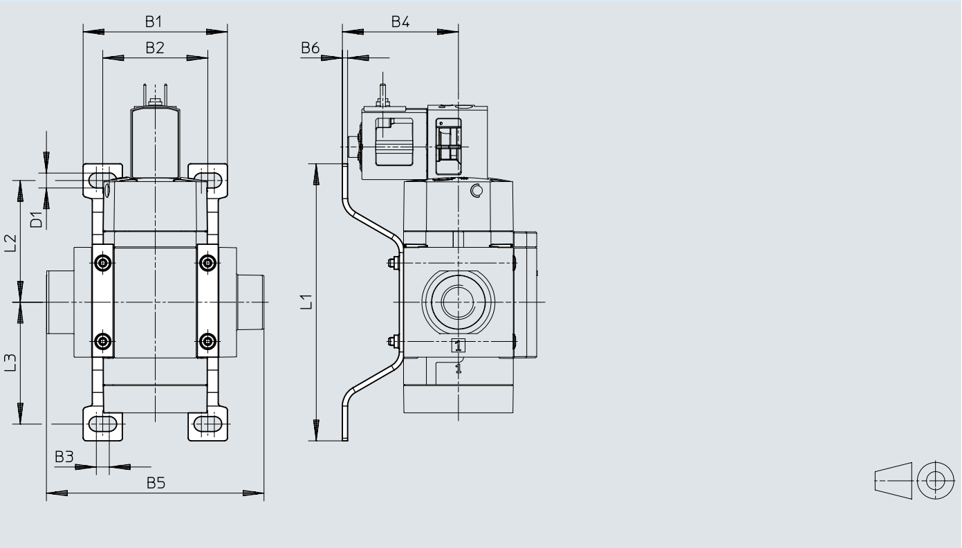
Dimensiones – Conjunto para el montaje en la pared MS...-WPE-B (accesorio)
