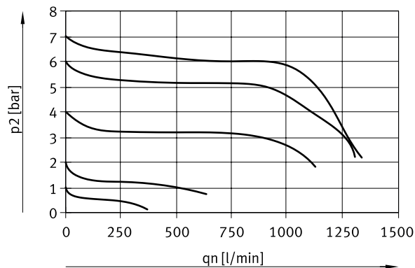
Caudal normal qn en función de la presión de salida p2 (MSB4-1/8; margen de regulación de presión 0,5 ... 12 bar; grado de filtración: 40 µm)
