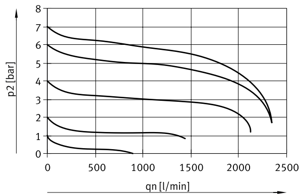
Caudal normal qn en función de la presión de salida p2 (MSB4-1/4; margen de regulación de presión 0,5 ... 12 bar; grado de filtración: 5 µm)
