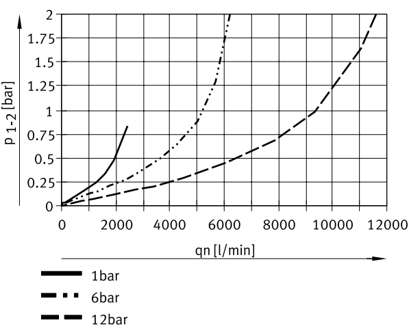
Caudal normal qn en función de la presión diferencial p1-2 (MS4-LOE-3/8)
