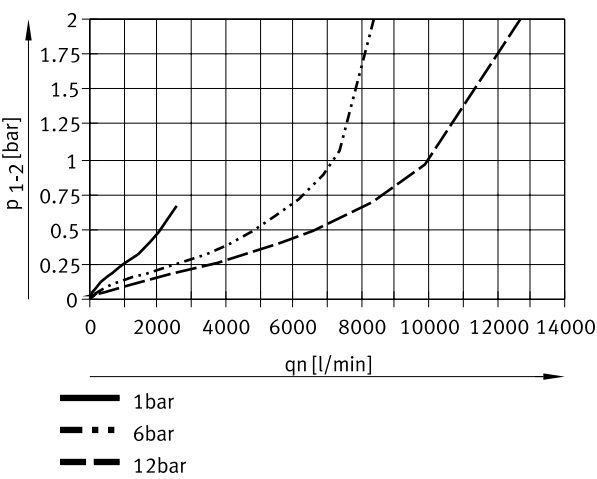
Caudal normal qn en función de la presión diferencial p1-2 (MS6-LOE-1/2)
