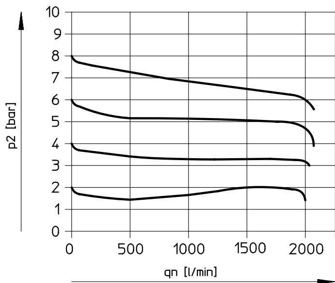
Caudal normal q_n en función de la presión de salida p_2 ( p_1 = 10 \text{ bar} ) – LR/LRS-1/4-D-MINI
