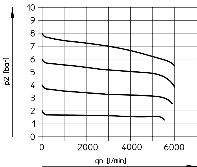
Caudal normal q_n en función de la presión de salida p_2 ( p_1 = 10 \text{ bar} ) – LR/LRS-1/2-D-MIDI
