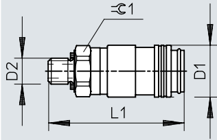
Dimensiones – Acoplamiento interior KD4, rosca exterior
