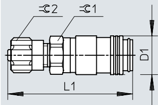
Dimensiones – Acoplamiento interior KD2, racor de unión rápida
