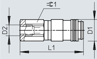
Dimensiones – Acoplamiento interior KD3, rosca interior
