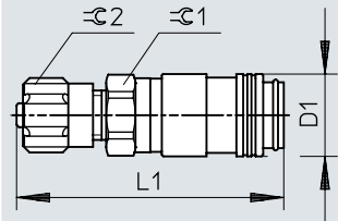
Dimensiones – Acoplamiento interior KD4, racor de unión rápida
