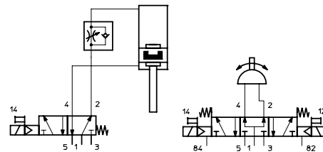
Esquema del circuito para HSP con módulo de posición de espera
