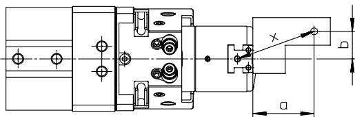
Fuerza de sujeción FH por mordaza a 0,6 MPa (6 bar, 87 psi) en función del brazo de palanca x y de la excentricidad a y b
