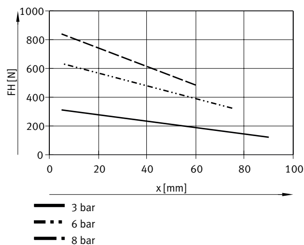
Fuerza de sujeción FH por mordaza en función de la presión de funcionamiento y del brazo de palanca x – Sujeción interior (abrir), de doble efecto – HGDD-63
