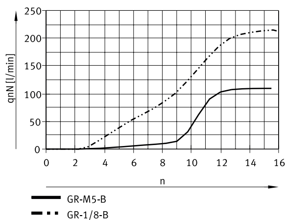
Caudal nominal normal qnN con 6 → 5 bar en función de las revoluciones del husillo n (GRO-M5-B, GRO-1/8-B)
