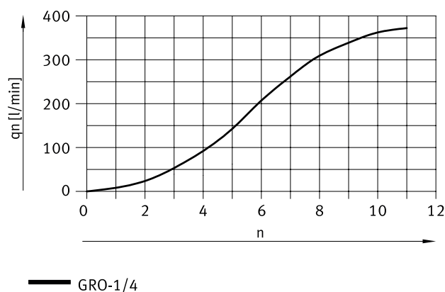
Caudal nominal normal qnN con 6 → 5 bar en función de las revoluciones del husillo n (GRO-1/4)
