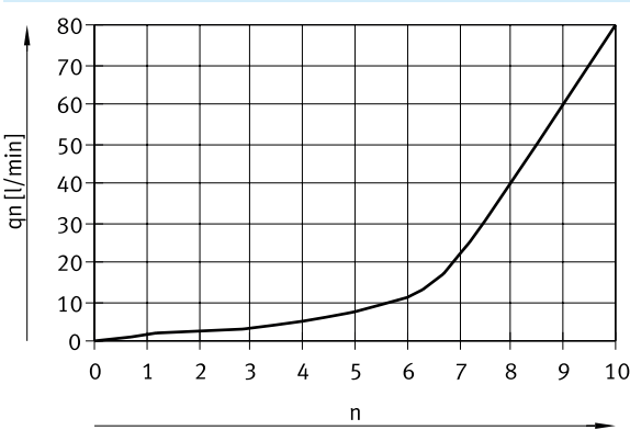
Caudal normal qn a 6 → 0 bar en función de las revoluciones del husillo n (GRLA/GRLZ-M5, Mini – racor QS, metal)
