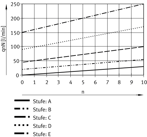
Caudal nominal normal qnN a 6 → 5 bar en función de la posición del tornillo control de servo (escala) (GRLSA-1/8 – racor QS, metal)
