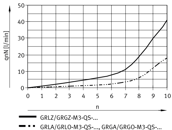
Caudal nominal normal q_{nN} a 6 → 5 bar en función de las revoluciones del husillo n (GRLA/GRLZ-M3, Mini – racor QS, metal)
