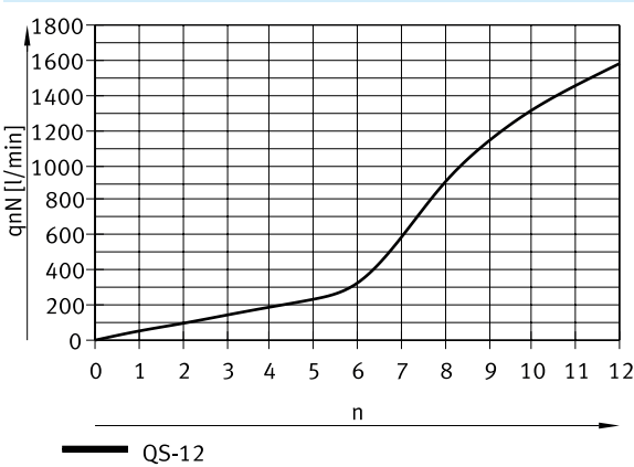
Caudal nominal normal qnN a 6 → 5 bar en función de las revoluciones del husillo n (GRLA/GRLZ-1/2 – racor QS, metal)
