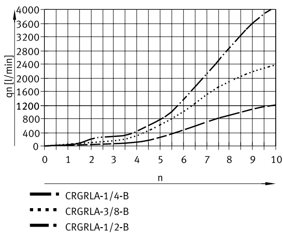
Caudal normal q_n a 6 \rightarrow 0 bar en función de las revoluciones del husillo n (CRGRLA-1/4, CRGRLA-3/8, CRGRLA-1/2 – rosca interior, acero inoxidable)
