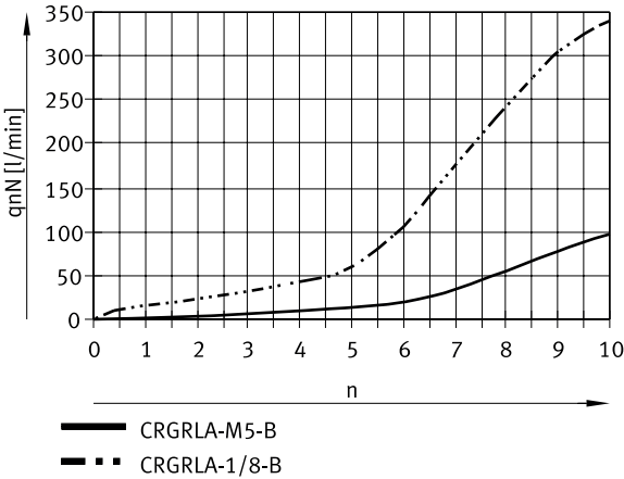
Caudal nominal normal qnN a 6 → 5 bar en función de las revoluciones del husillo n (CRGRLA-M5, CRGRLA-1/8 – rosca interior, acero inoxidable)
