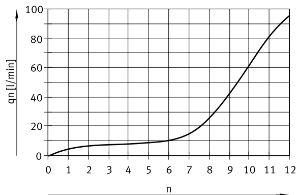
Caudal normal q_n a 6 → 0 bar en función de las revoluciones del husillo n (GRLA/GRLZ-M3, Mini – racor QS, metal)
