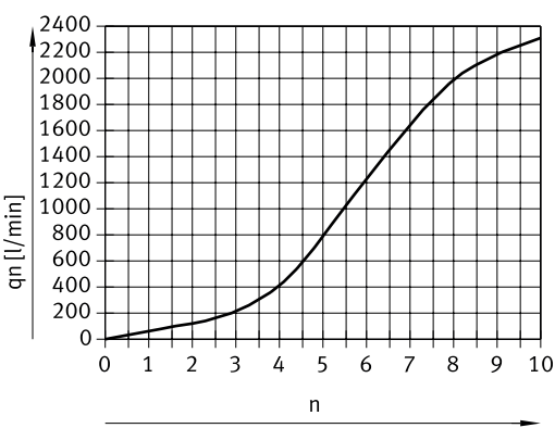
Caudal normal qn a 6 → 0 bar en función de las revoluciones del husillo n (GRLA/GRLZ-3/8 – rosca interior/boquilla estriada, metal)
