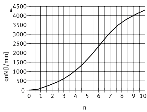
Caudal nominal normal qnN a 6 → 5 bar en función de las revoluciones del husillo n (GRLA/GRLZ-3/4 – rosca interior/boquilla estriada, metal)
