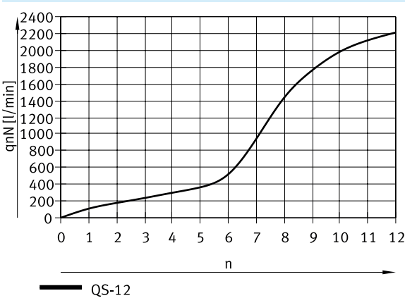
Caudal normal qn a 6 → 0 bar en función de las revoluciones del husillo n (GRLA/GRLZ-1/2 – racor QS, metal)
