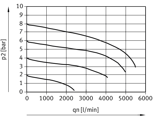
Caudal normal qn en función de la presión de salida p2 (FRC-1/2-D-MIDI)
