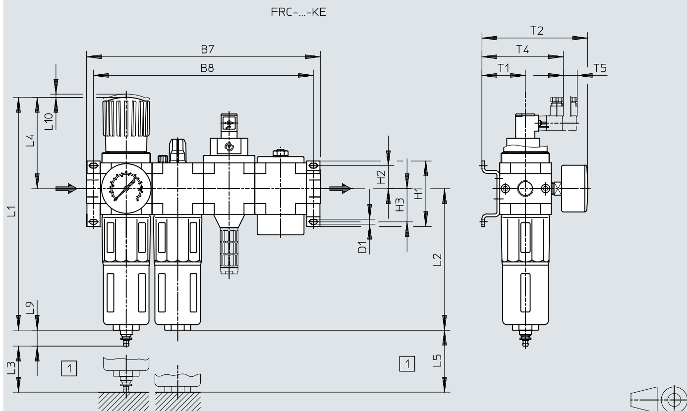
[1] Medidas de instalación
