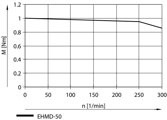
Para rotación: momento de giro M en función de las revoluciones n para EHMD-50
