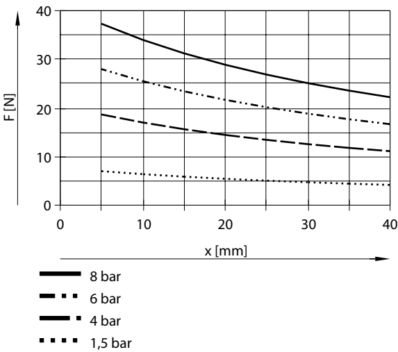
Para agarre, neumático: fuerza de sujeción F en función del brazo de palanca x y de la presión de funcionamiento d para EHMD-40
