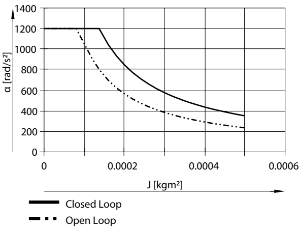
Para rotación: aceleración angular en función del momento de inercia J para EHMD-40
