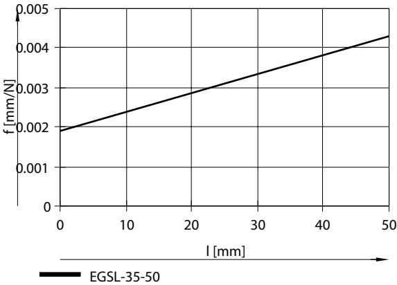
Desviación x en función de la fuerza Fz para tamaño 35
