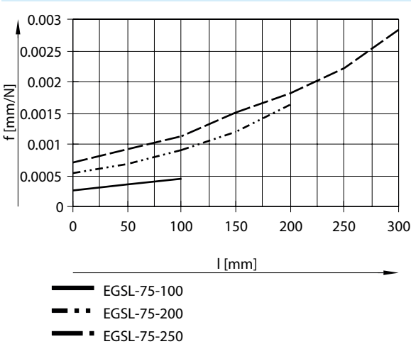
Desviación x en función de la fuerza Fy para tamaño 75
