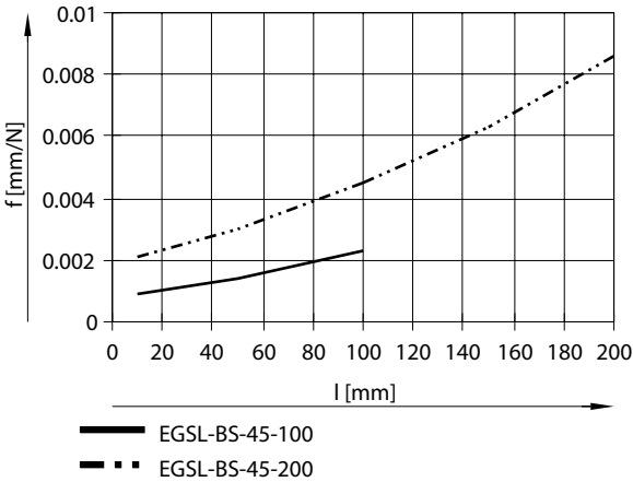
Desviación x en función de la fuerza Fz para tamaño 45
