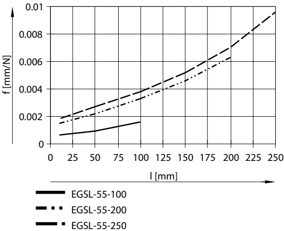
Desviación x en función de la fuerza Fz para tamaño 55
