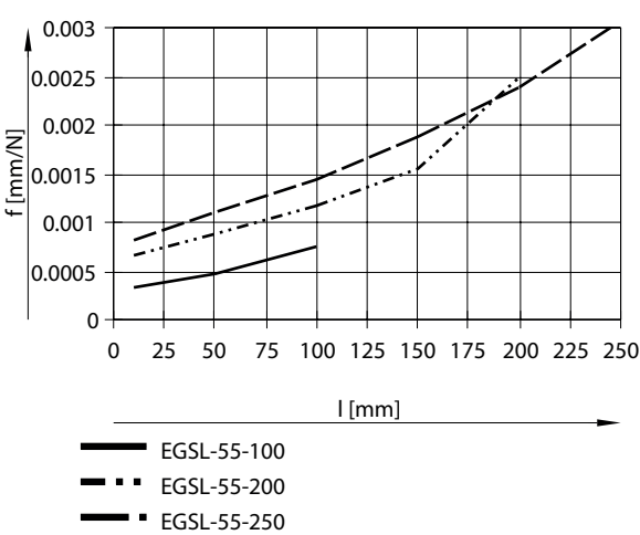
Desviación x en función de la fuerza Fy para tamaño 55
