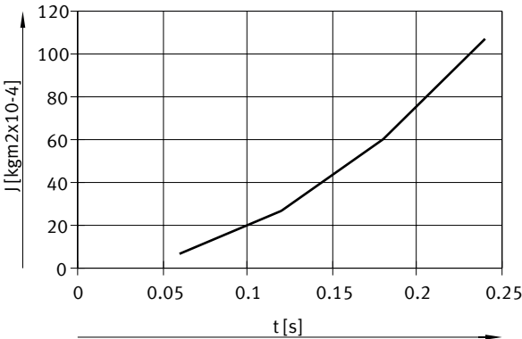
Tiempos necesarios de apertura y cierre T a 0,6 MPa (6 bar, 87 psi) en función del momento de inercia de la masa de los dedos de sujeción – DHWS-40
