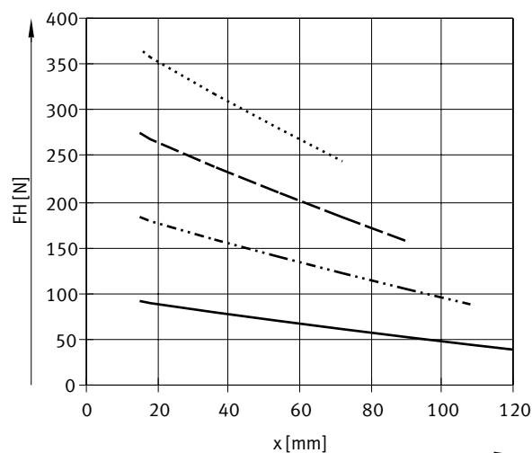
Fuerza de sujeción FH por mordaza en función de la presión de funcionamiento y del brazo de palanca x – Sujeción interior (abrir), de doble efecto – DHDS-50
