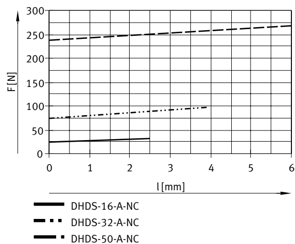
Fuerza del muelle FF en función del tamaño y de la carrera de las mordazas l – Con aseguramiento de la fuerza de sujeción para DHDS-...-NC
