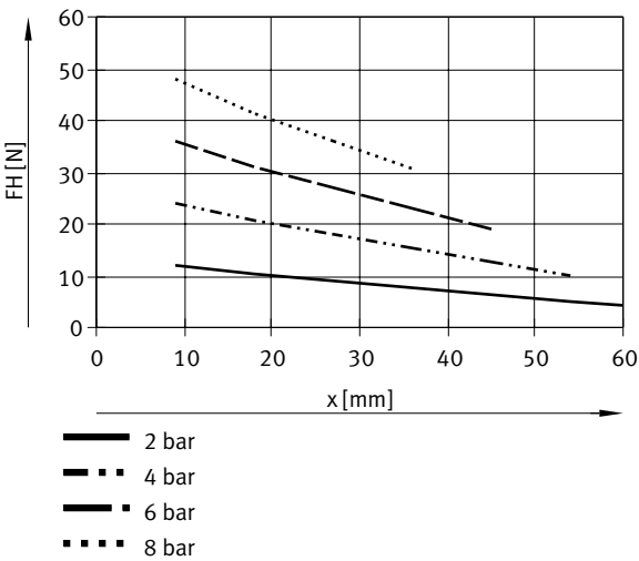
Fuerza de sujeción FH por mordaza en función de la presión de funcionamiento y del brazo de palanca x – Sujeción interior (abrir), de doble efecto – DHDS-16
