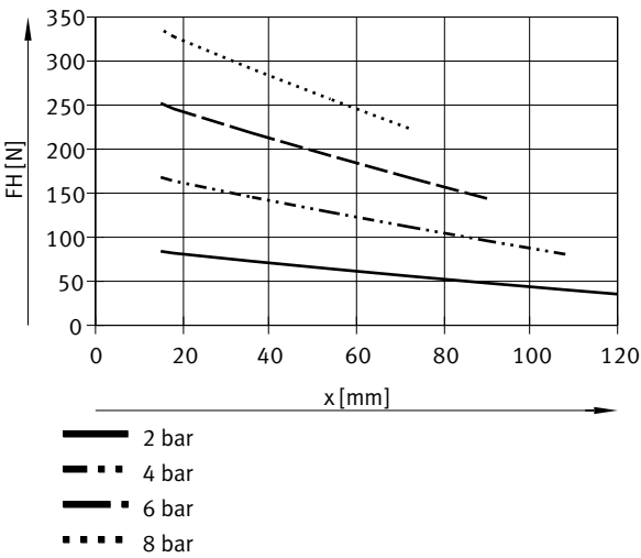
Fuerza de sujeción FH por mordaza en función de la presión de funcionamiento y del brazo de palanca x – Sujeción externa (cerrar), de doble efecto – DHDS-50
