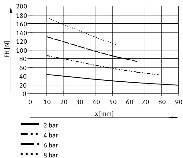
Fuerza de sujeción FH por mordaza en función de la presión de funcionamiento y del brazo de palanca x – Sujeción interior (abrir), de doble efecto – DHDS-32
