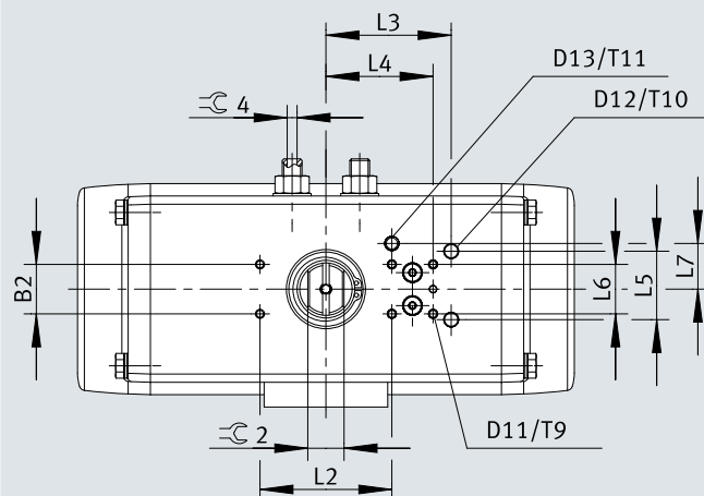
Dimensiones – DFPD-C de efecto simple, tamaño 20 ... 480, variante VDE2
