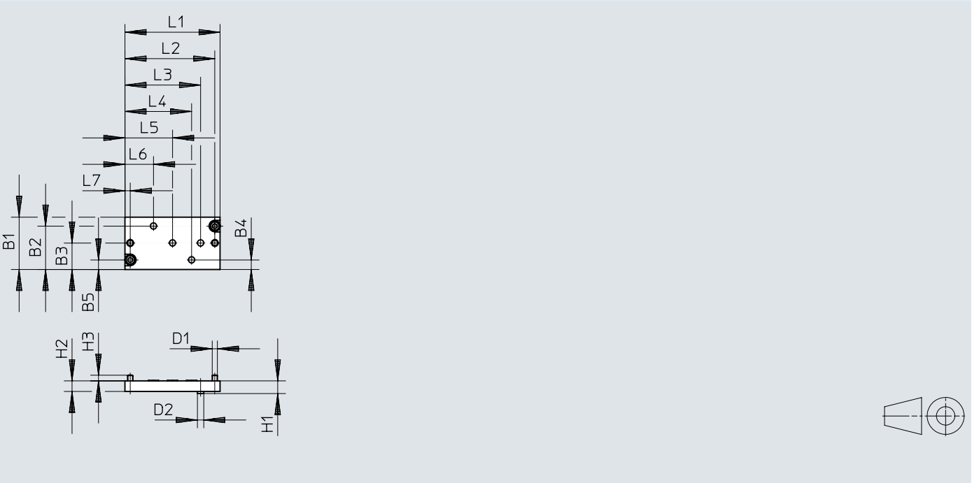
Dimensiones – Kit adaptador DADG-AK-F9-1
