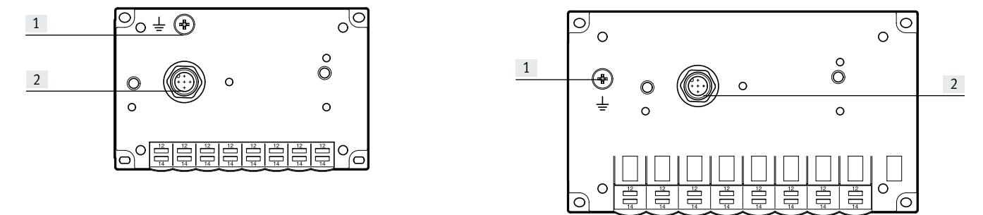
[1] Tornillo de puesta a tierra [2] Interfaz I-Port/IO-Link [1] Tornillo de puesta a tierra [2] Interfaz I-Port/IO-Link
