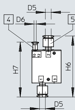
CPE18-...-QS-10
