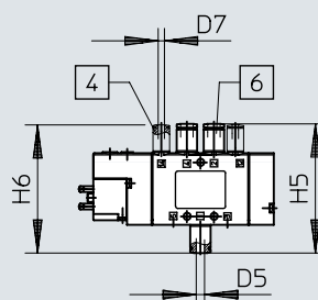
CPE10-...-QS-4
