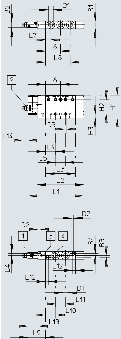
CPE 14-M1CH-5L...
