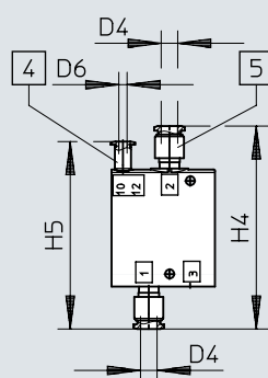
CPE18-...-QS-8
