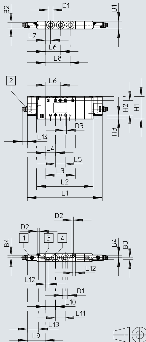
CPE 14-M1...H-5/3-...
