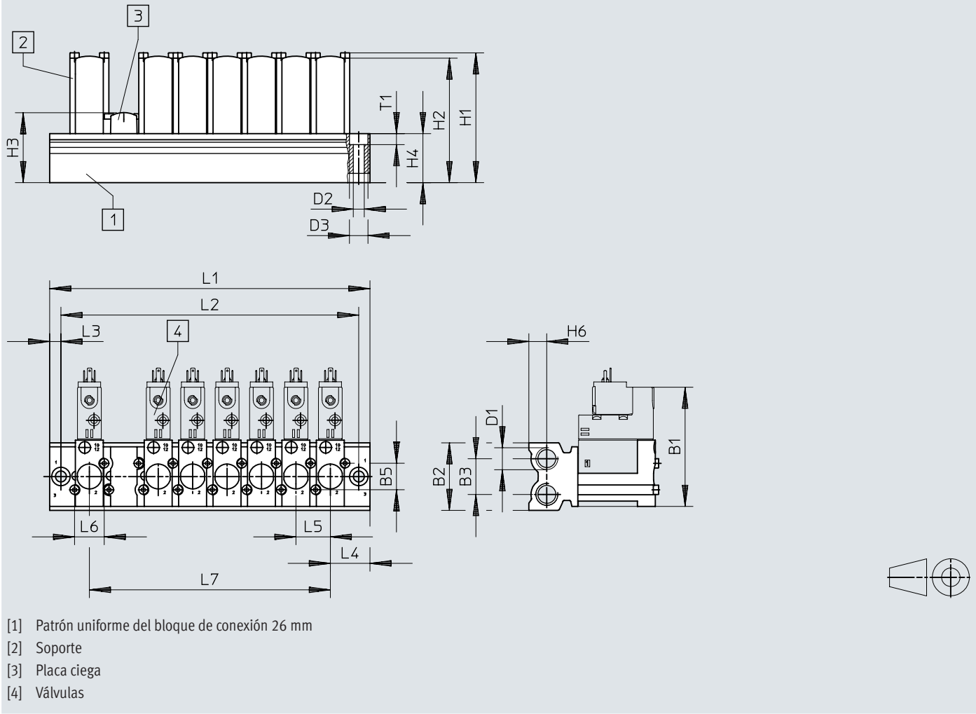
Dimensiones – CPE18, bloque de conexión, batería de patrón fijo 3/2
