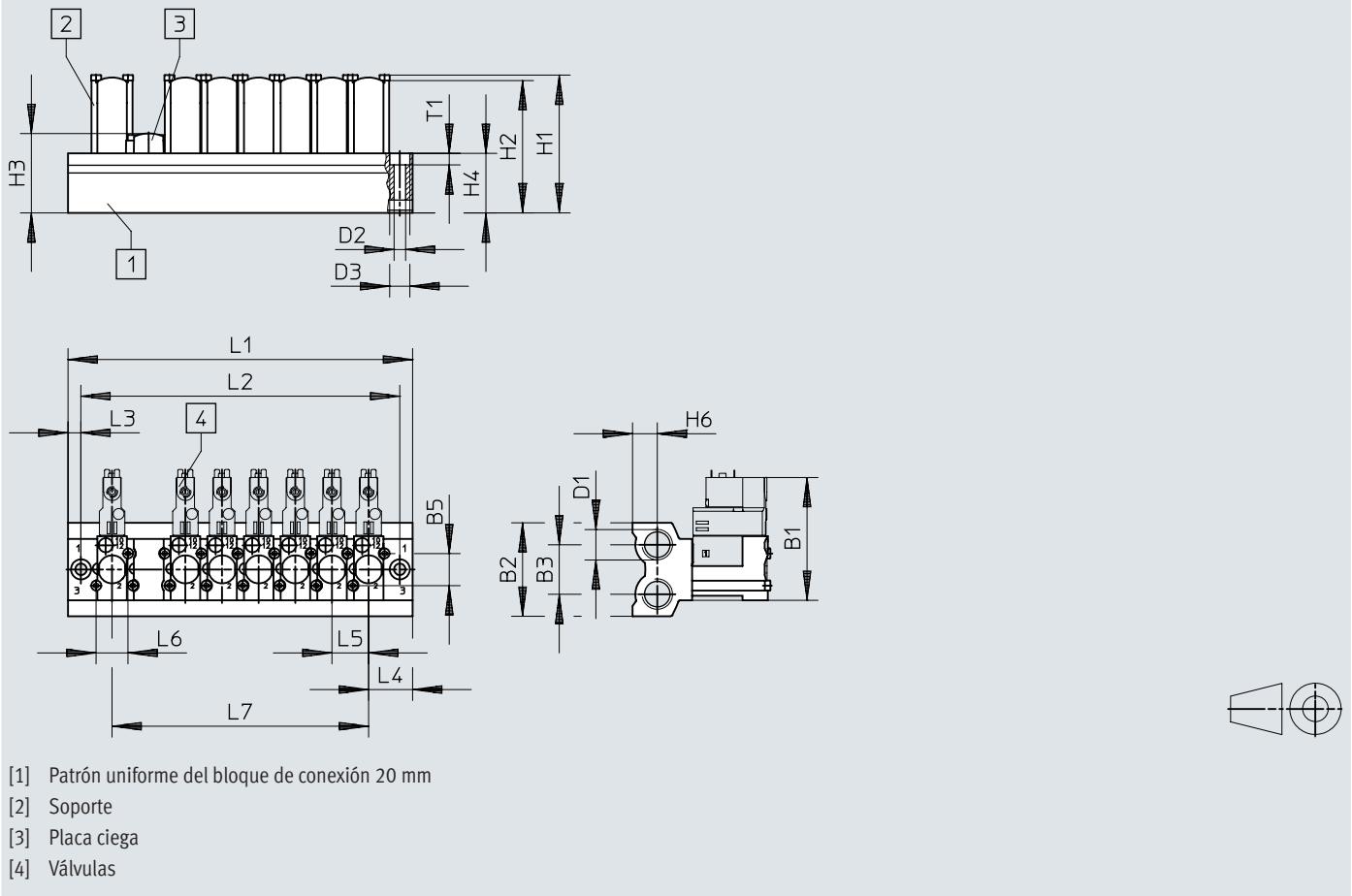
Dimensiones – CPE14, bloque de conexión, batería de patrón fijo 3/2
