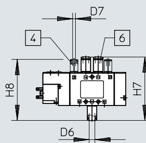
CPE10-...-QS-6
