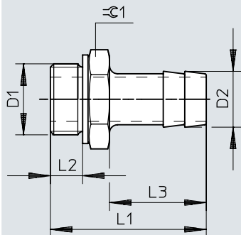
Dimensiones – Boquilla para tubos N-...-P-...-MS
