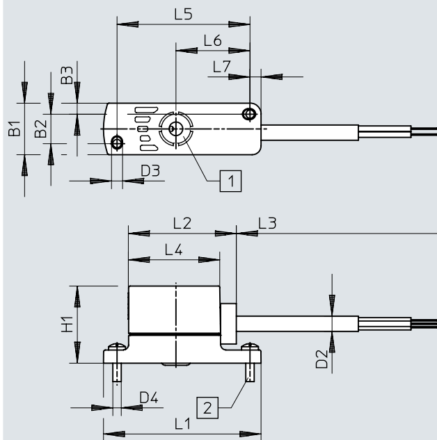
Dimensions – SPTE-...-F
