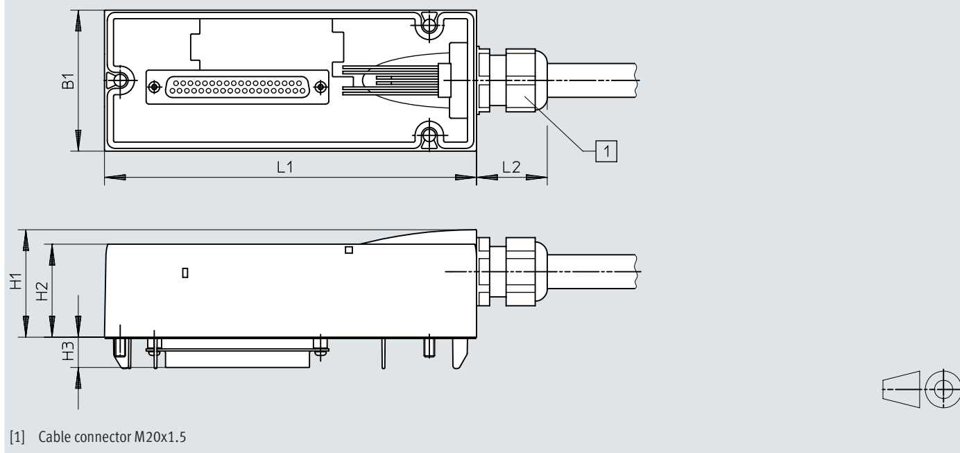
Dimensions – NEBV-S1W37
