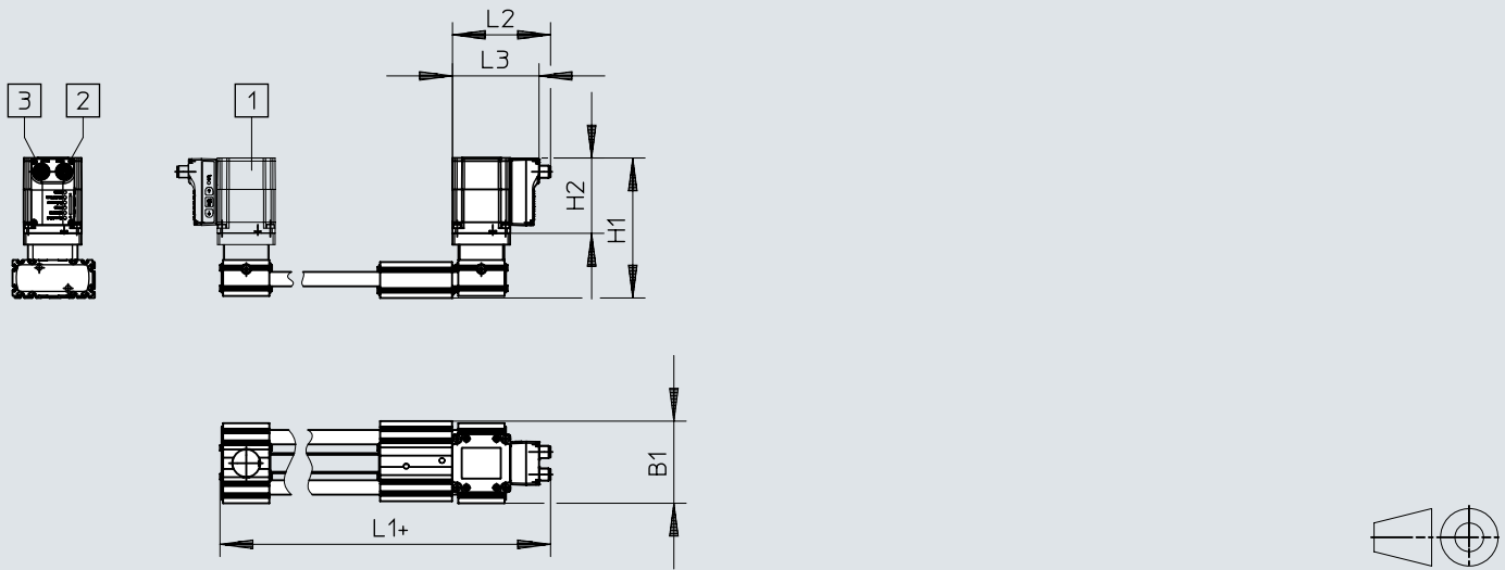
Dimensions – ELGE-...-AR/AL
