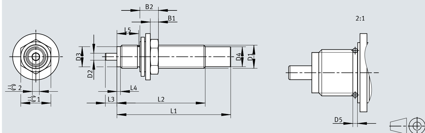
Dimensions – Shock absorber DYSD-Q13-...
