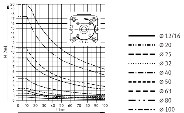
Drehmoment M in Abhängigkeit von der Hublänge l
