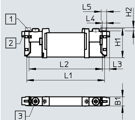
[1] Elektrischer Anschluss vertikal
