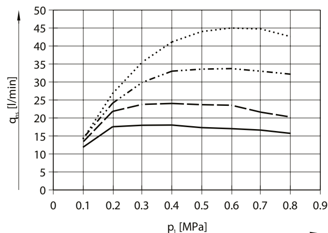
Saugvolumenstrom q_{vs} in Abhängigkeit vom Arbeitsdruck p_1
