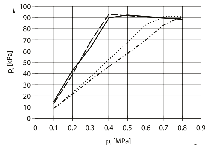
Vakuum p_u in Abhängigkeit vom Arbeitsdruck p_1
